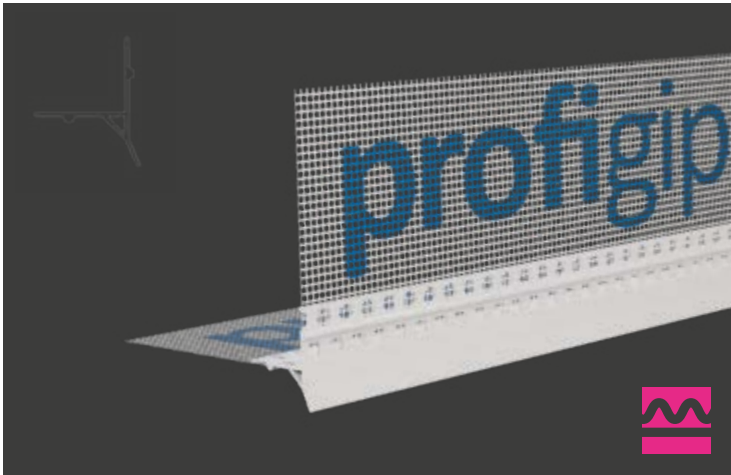
Profil okapowy podtynkowy LTD Underplaster PVC profile with eaves LTD Капельник ЛТД Profil PVC cu picurator acoperit LTD
