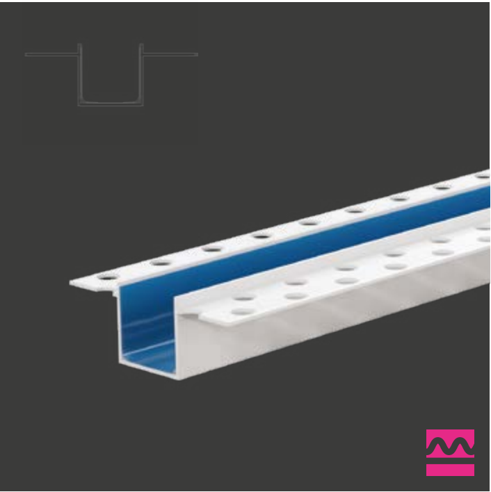
Listwa PCV do boniowania Corner bead for rustication Рустовочный профиль ПВХ Profil PVC pentru ornamentare rustica
