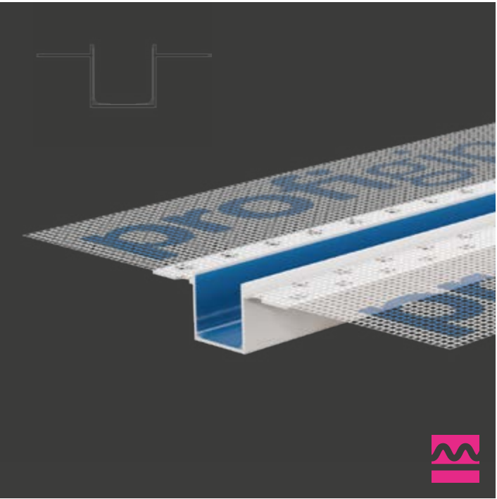
Listwa PCV do boniowania z siatką Corner bead for rustication with mesh Рустовочный профиль ПВХ с сеткой Profil PVC pentru ornamentare rustica cu plasa
